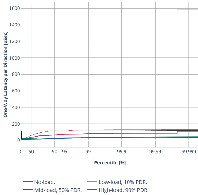
Latency: rdma-ethip6-ip6base
