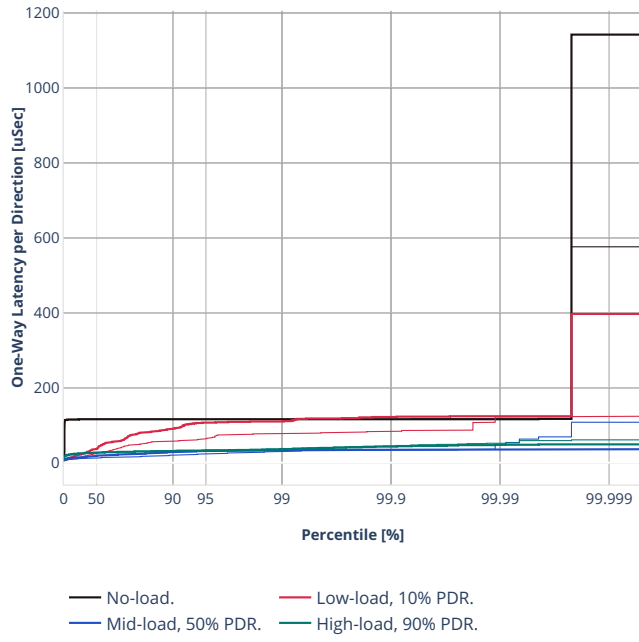
Latency: rdma-ethip4-ip4scale20k
