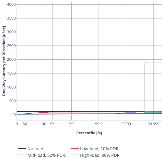
Latency: rdma-ethip4-ip4base
