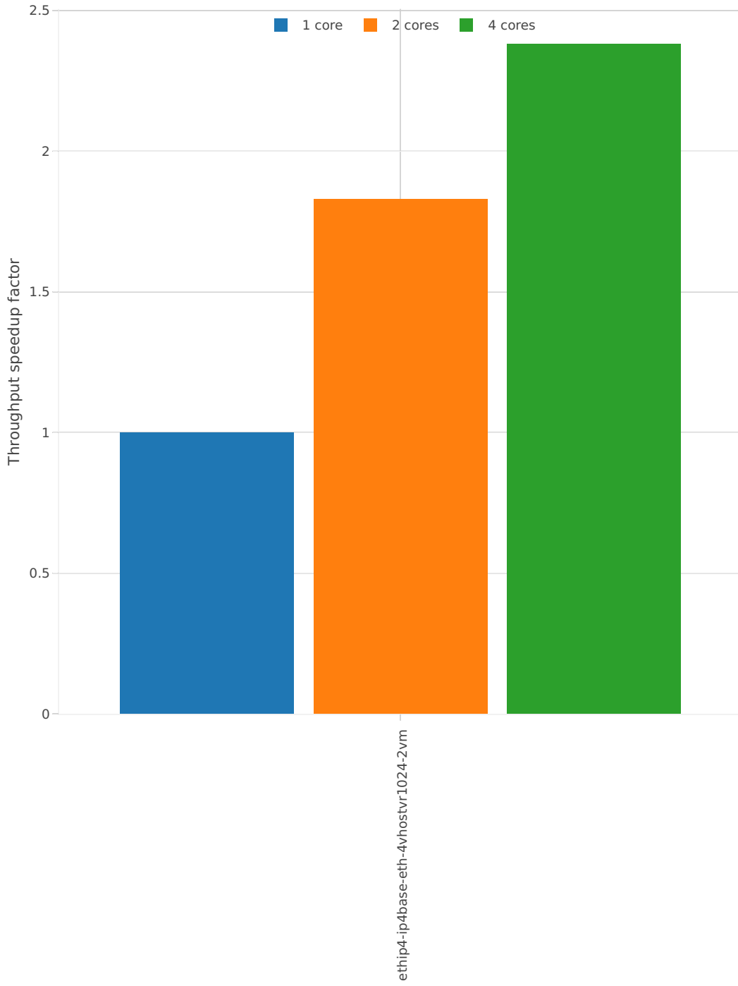
64B-*,*vhost.*-ndrdisc
